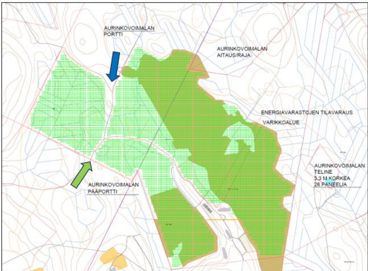
Kuva 2. Alustava paneelilayout ja ajoportit (nuolet) alueelle (Liite 3). Pääportti vihreällä
